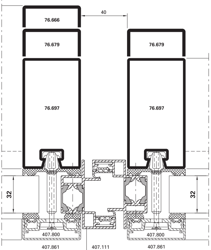
Situation de montage profilés de feuilure dans VISS TV
