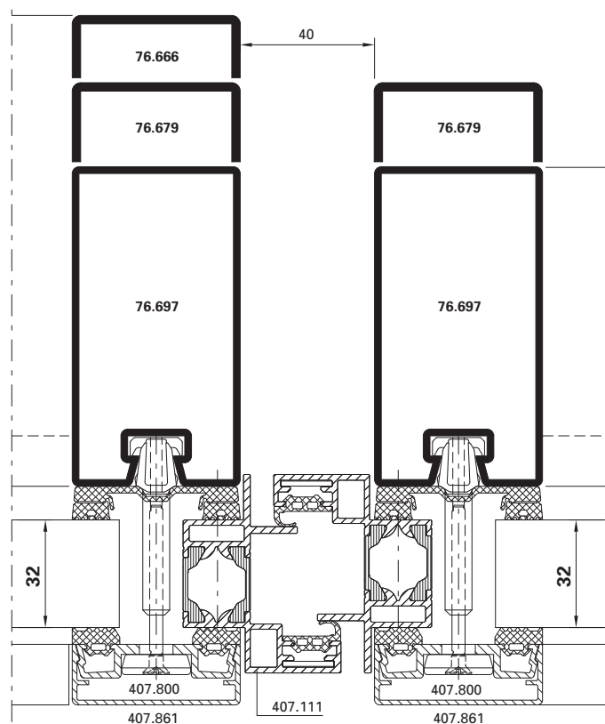
Situation de montage profilés de feuillure dans VISS TVS
